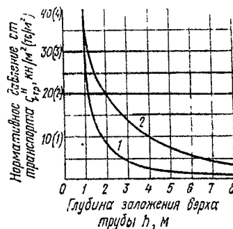
Рис. 1. Зависимость нормативного равномерно распределенного давления транспорта q_{тр}^н от глубины заложения трубопровода
